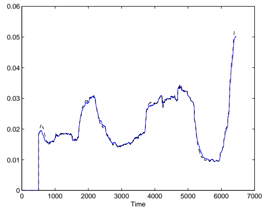
(d) \text{vol}(\text{JPM})(t) (—) and 20 days forecasting (---)
